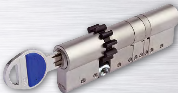
OBOUSTRANNÁ CYLINDRICKÁ VLOŽKA TOKOZ TECH S PASTORKEM (DESETIZUBÉ KOLEČKO)
